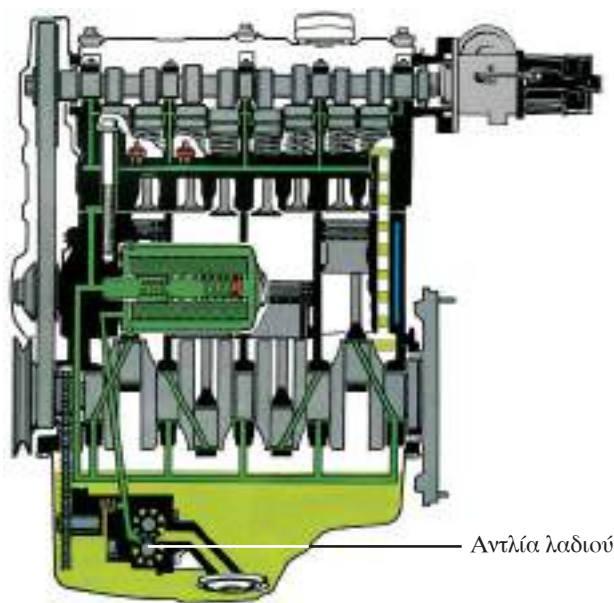
Σχ. 3 Σύστημα λίπανσεως.
